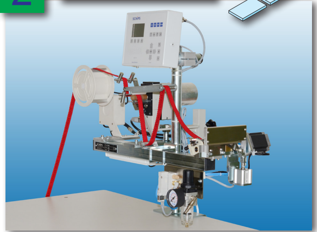
Bandablängautomat kompakt und preisgünstig
