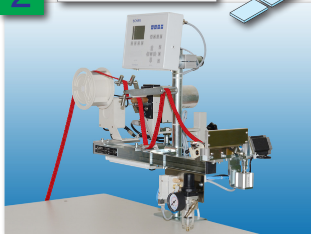
Automático de corte de cinta, compacto y de bajo coste
